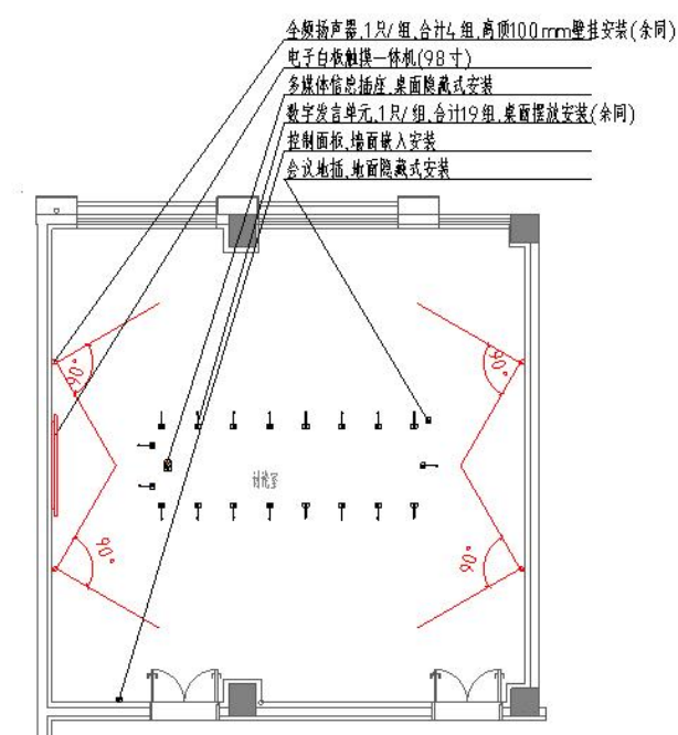
图3-17：大讨论室布置图
