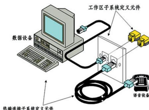
图3-6：工作区子系统示意图
