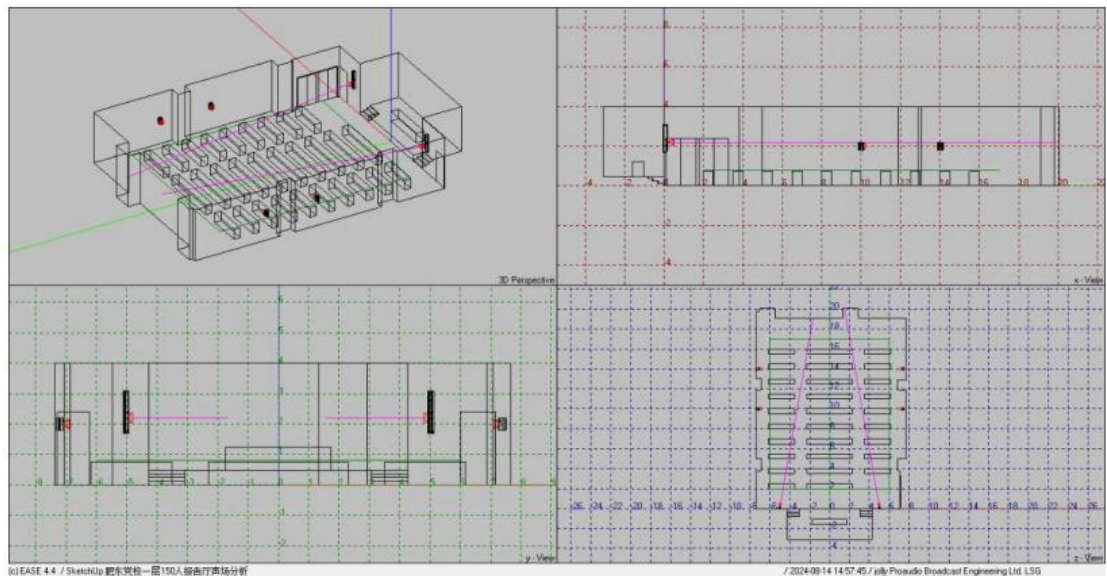
图3-16：150人报告厅音箱指向图
