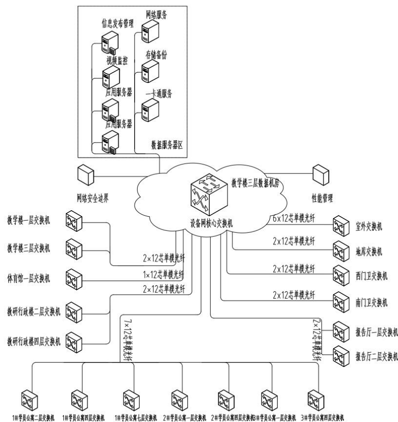
图3-4：设备网网络拓扑图
