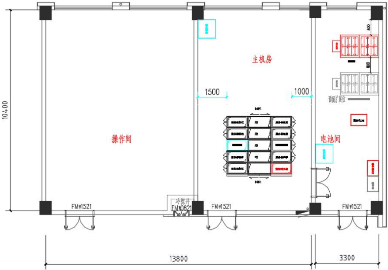
图3-13：弱电机房平面布置图
