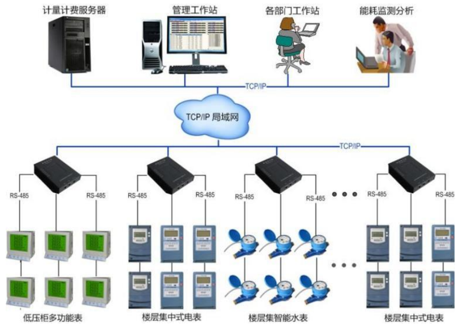
图3-24：能耗监控系统图
