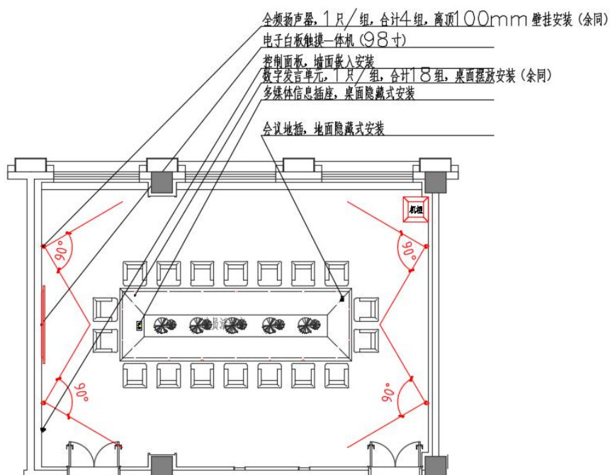
图3-19：大会议室布置图
