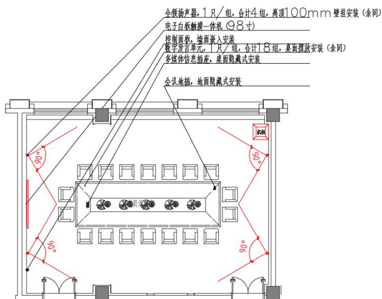
图3-18：党员活动室布置图
